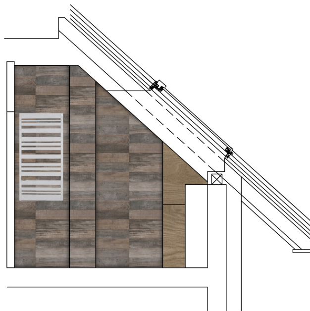
widok D/1:50
