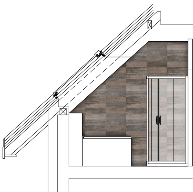
widok B/1:50
