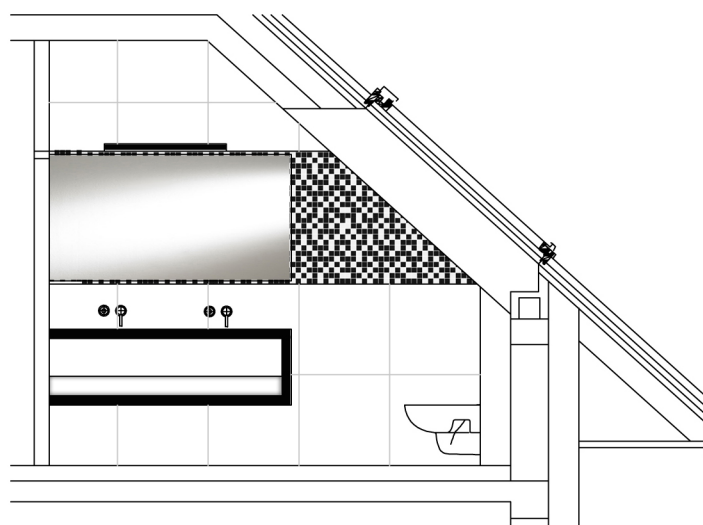
widok C/1:50
