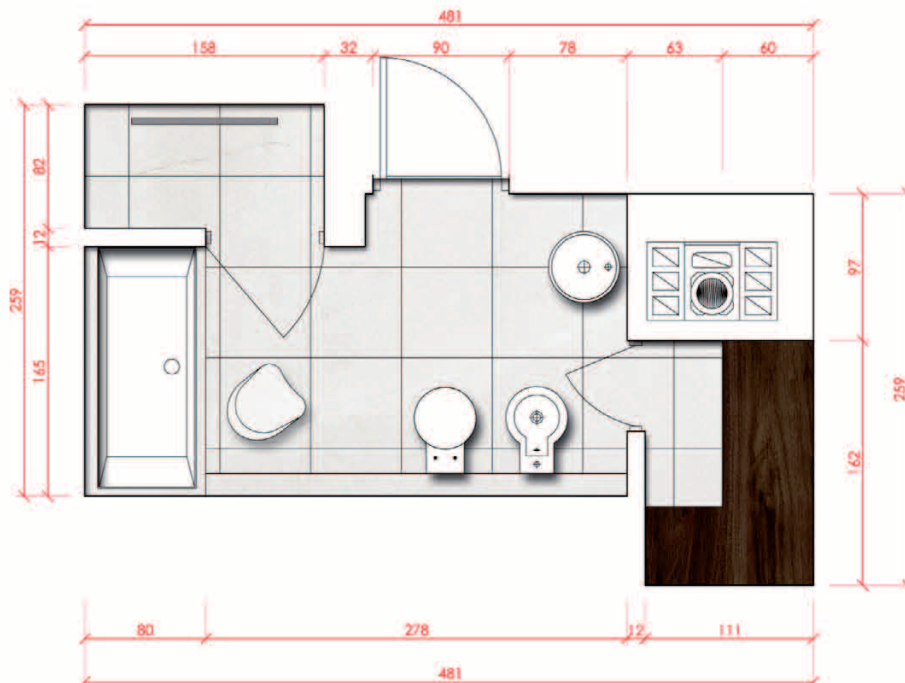
rzut/1:50
