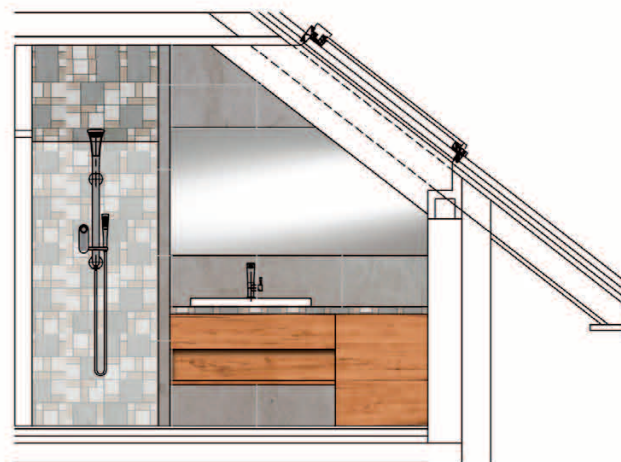
widok C/1:50
