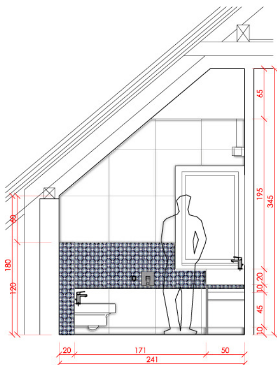
widok D/1:50
