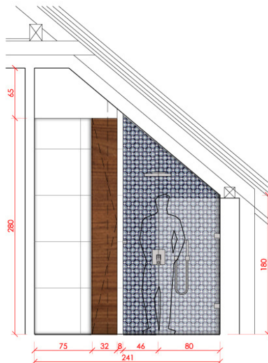
widok B/1:50
