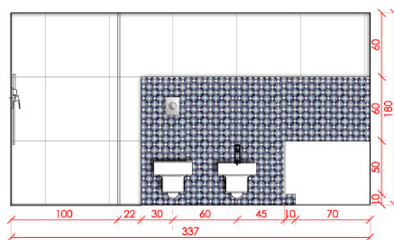
widok C/1:50
