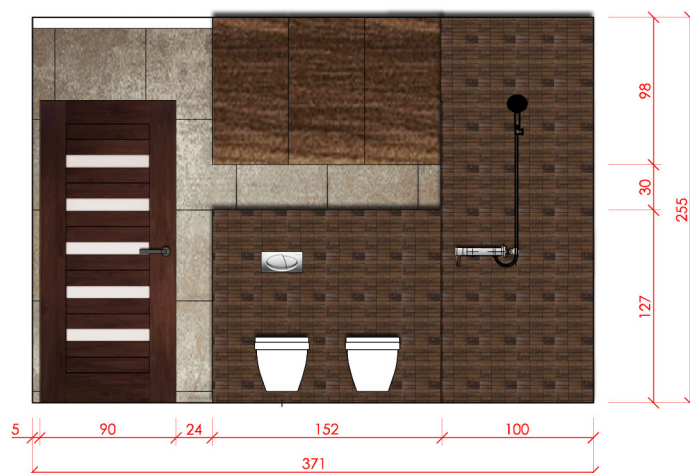
widok D/1:50
